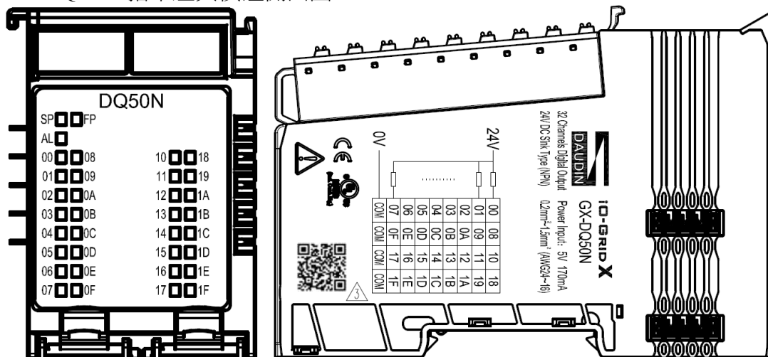
圖 4.13 GX-DQ50N 圖面
