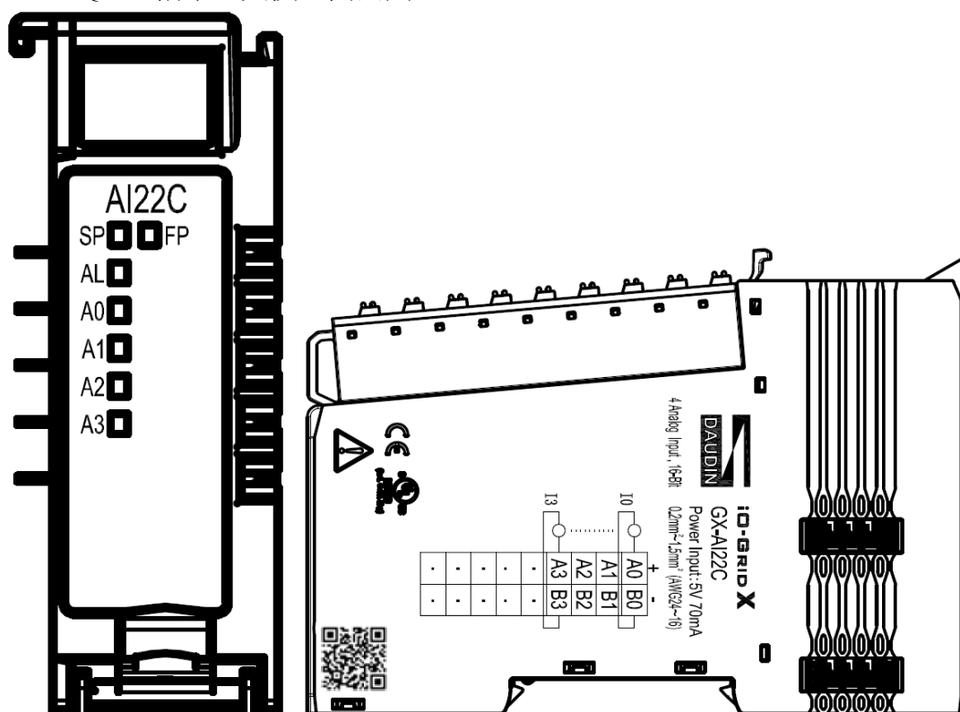
圖 4. 28 GX-AQ22C 圖面
