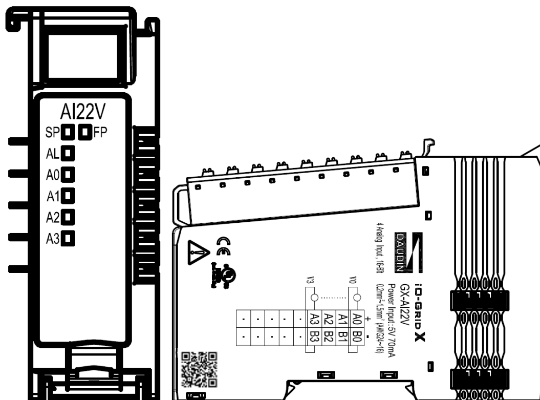
圖 4. 19 GX-AI22V 圖面
