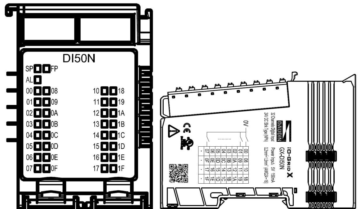
圖 4.7 GX-DI50N 圖面
