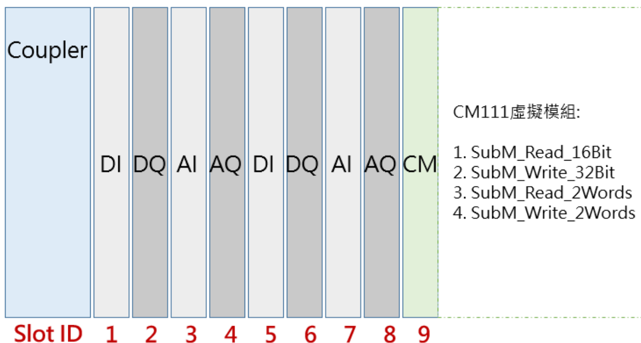
圖 9.11 模擬系統配置模組之組態圖
