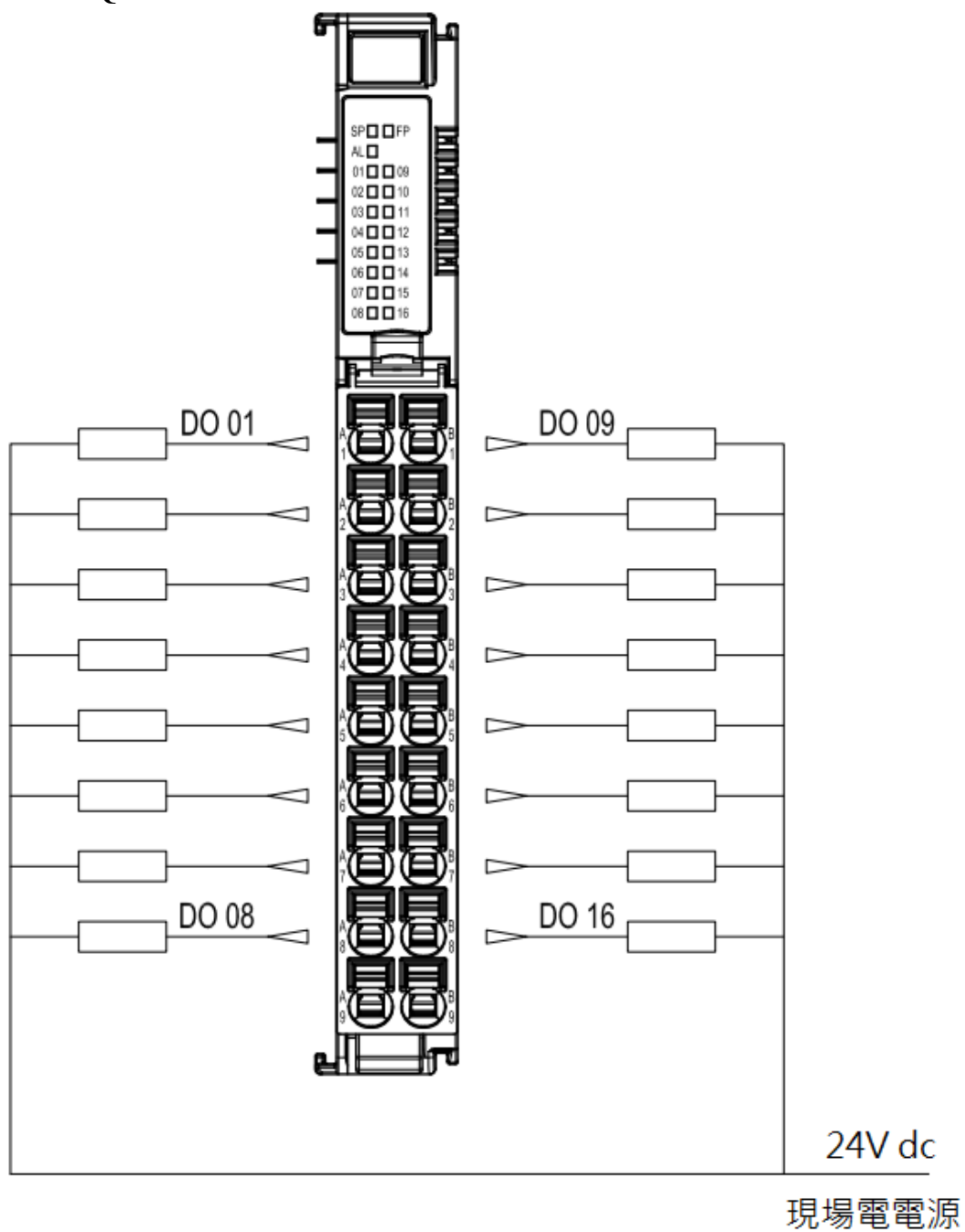
圖 8.8 GX-DQ40N 接線圖
