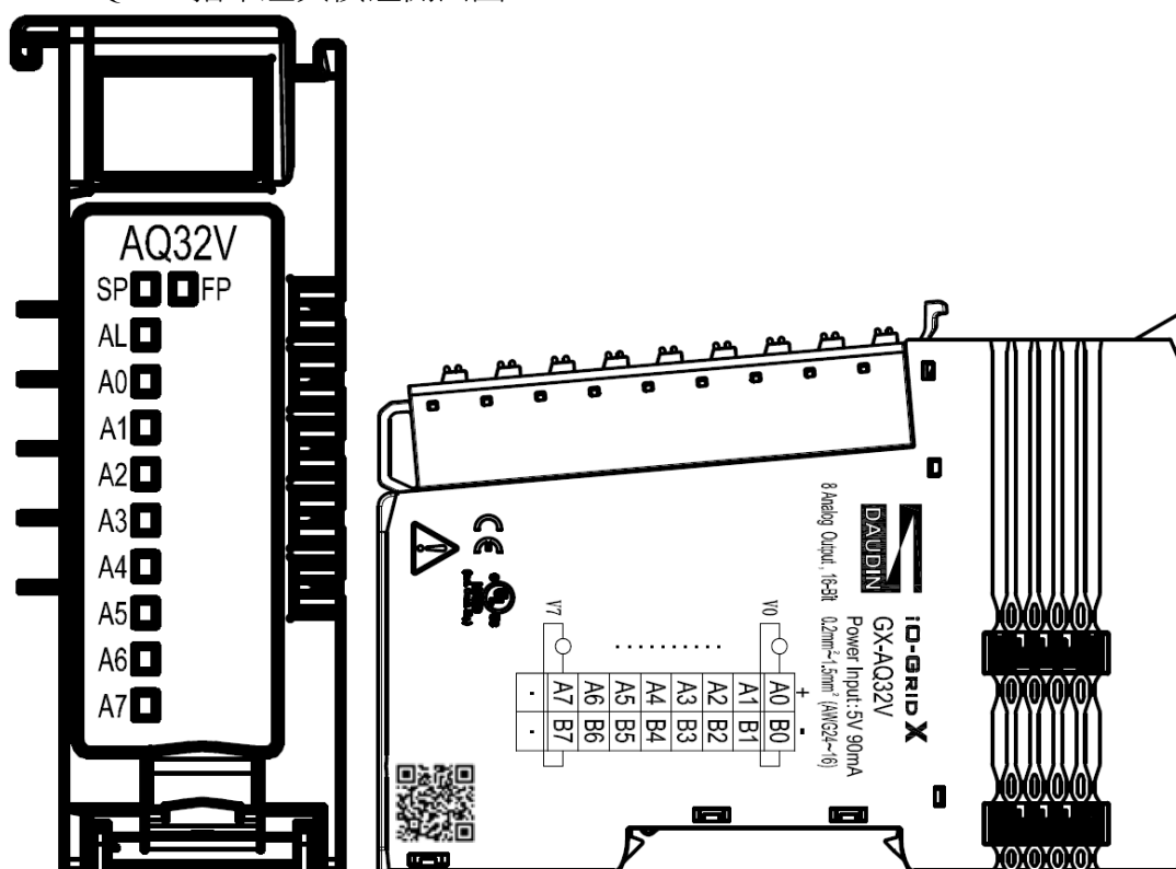
圖 4.31 GX-AQ32V 圖面
