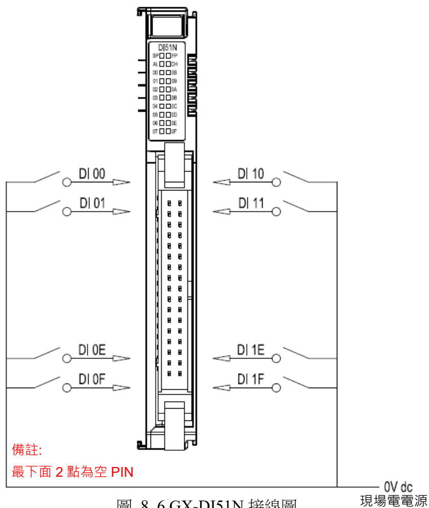
圖 8.6 GX-DI51N 接線圖
