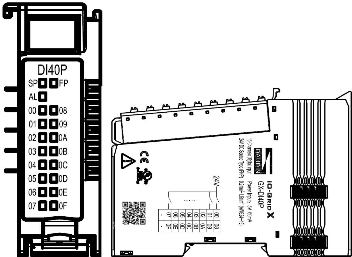
圖 4.5 GX-DI40P 圖面
